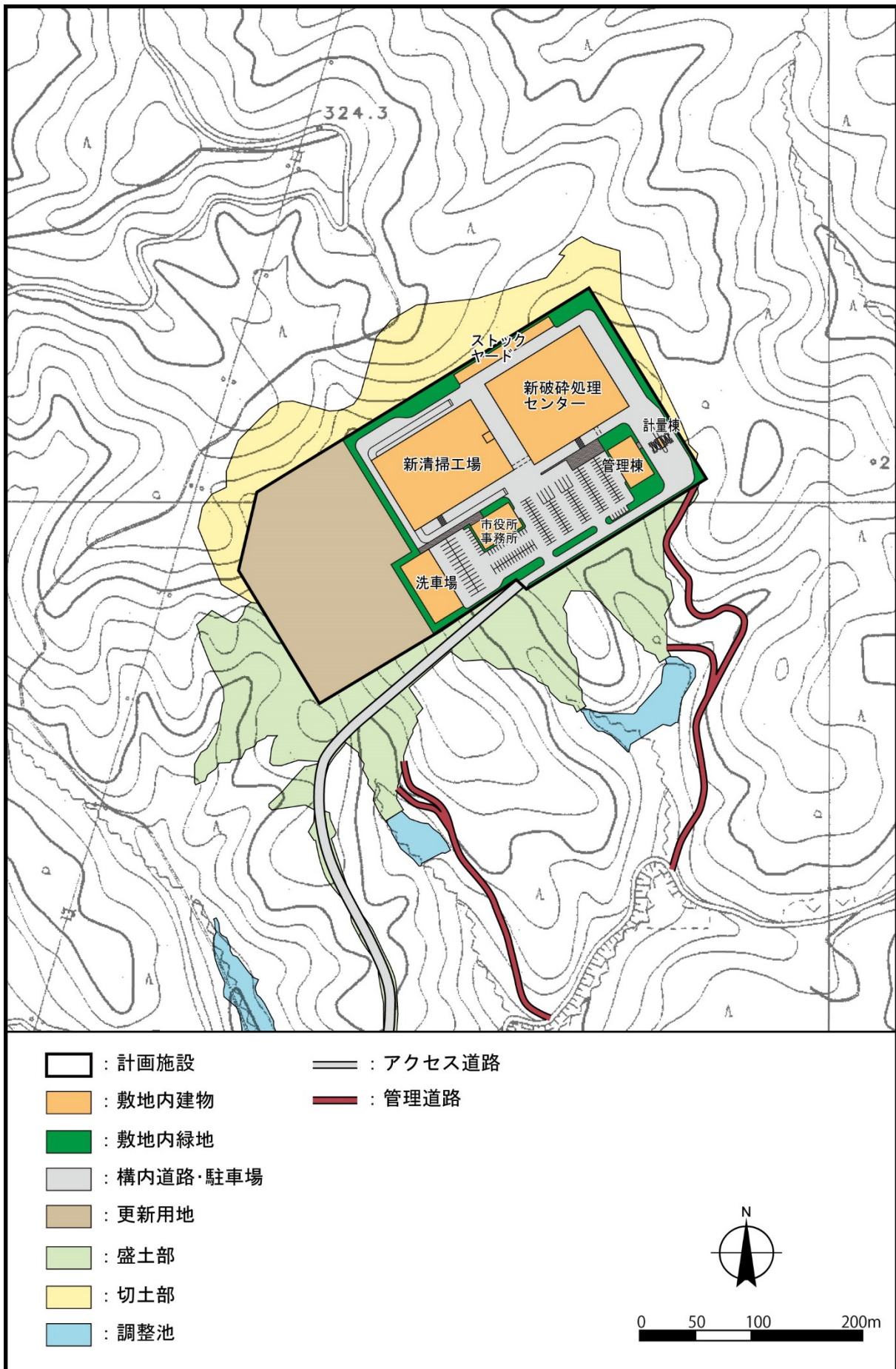
図 1-2 敷地造成及び施設配置計画
