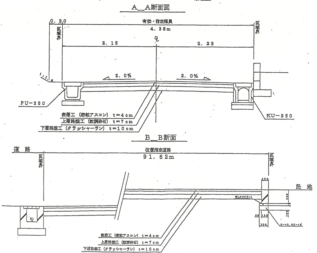
断面図 S=1/50
