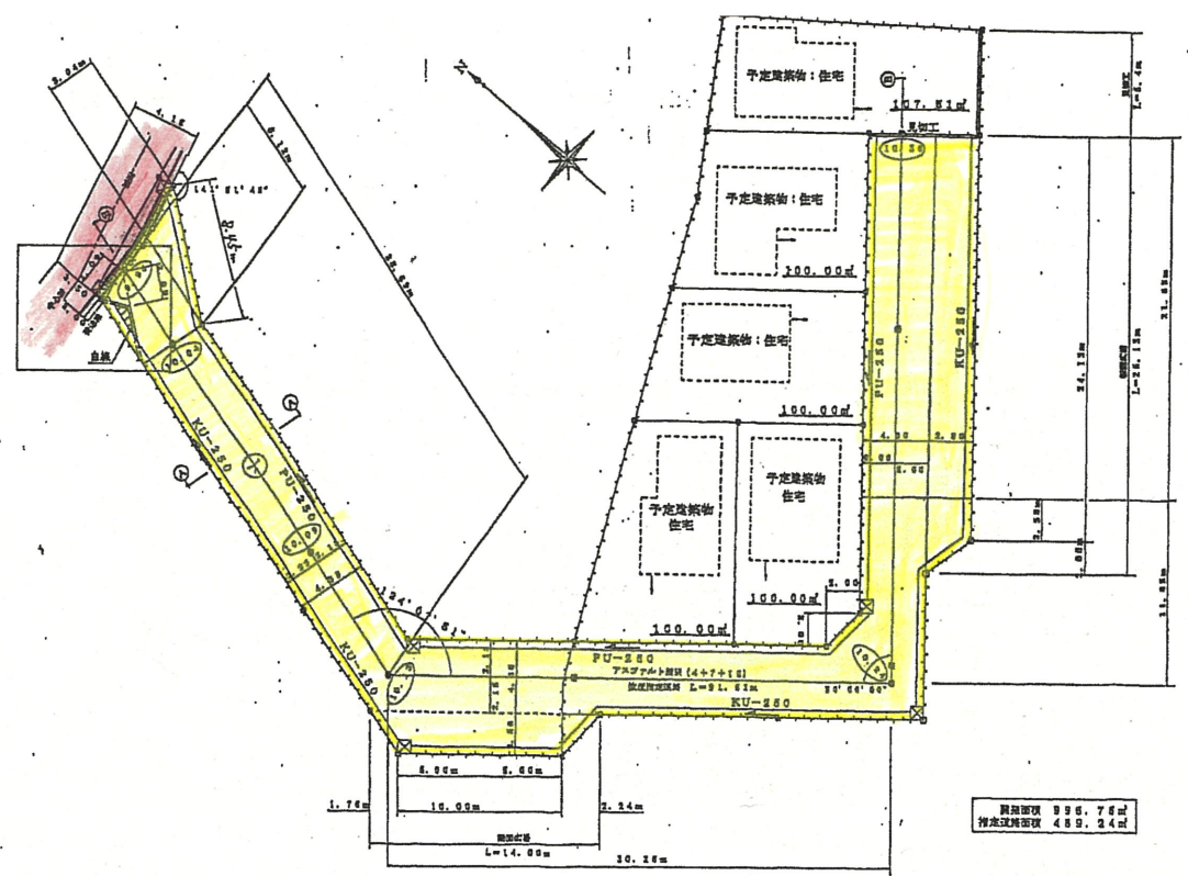
平面図 S=1/500
