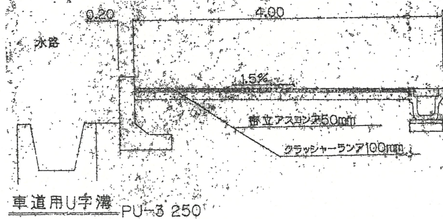
断面図 S = 1 / 50
