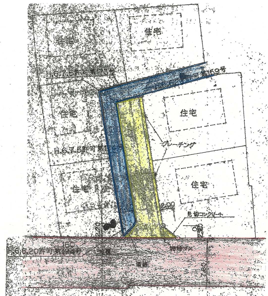
平面図 S = 1 / 300
