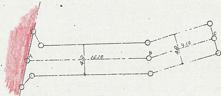
平面図 S = 1 / 300
