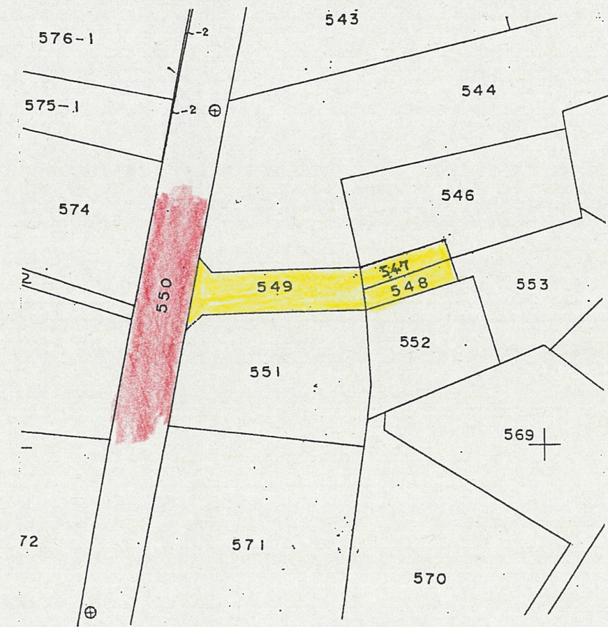
公図写 S = 1 / 500
