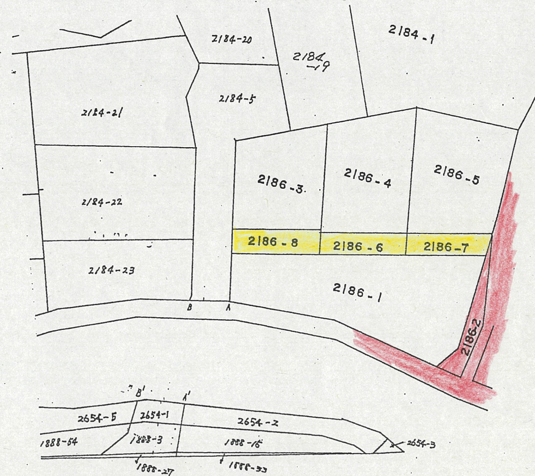
公図写 S = 1 / 600
