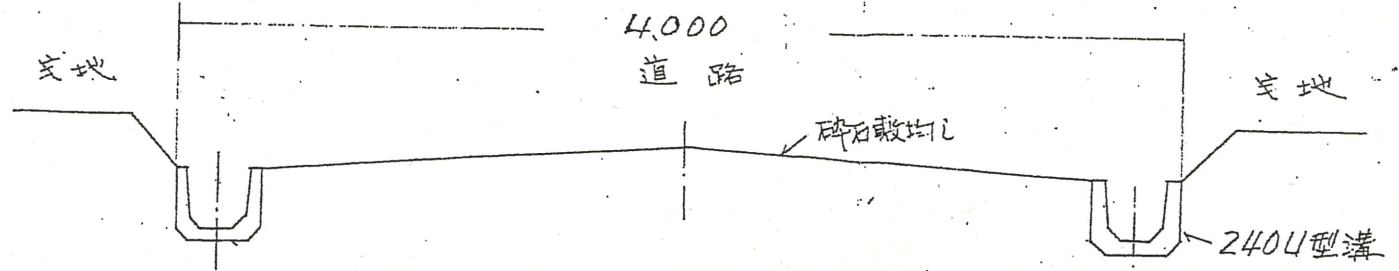
断面図 S = 1 / 30
