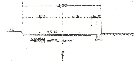
断面図 S = 1 / 100
