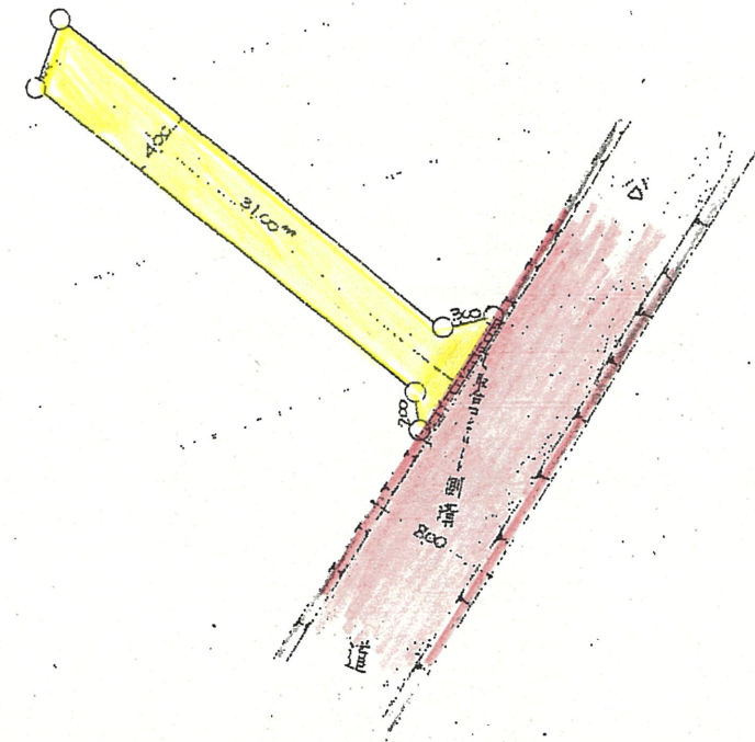
平面図 S = 1 / 500
