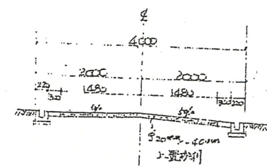
断面図 S = 1 / 100
