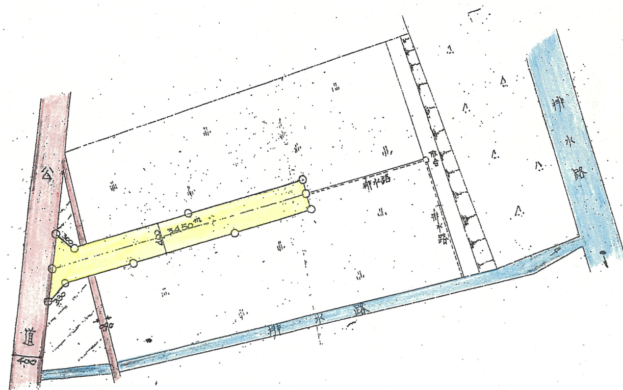
平面図 S = 1 / 500
