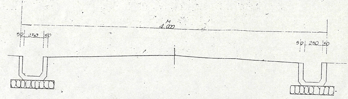
道路断面図 縮尺：1/30
