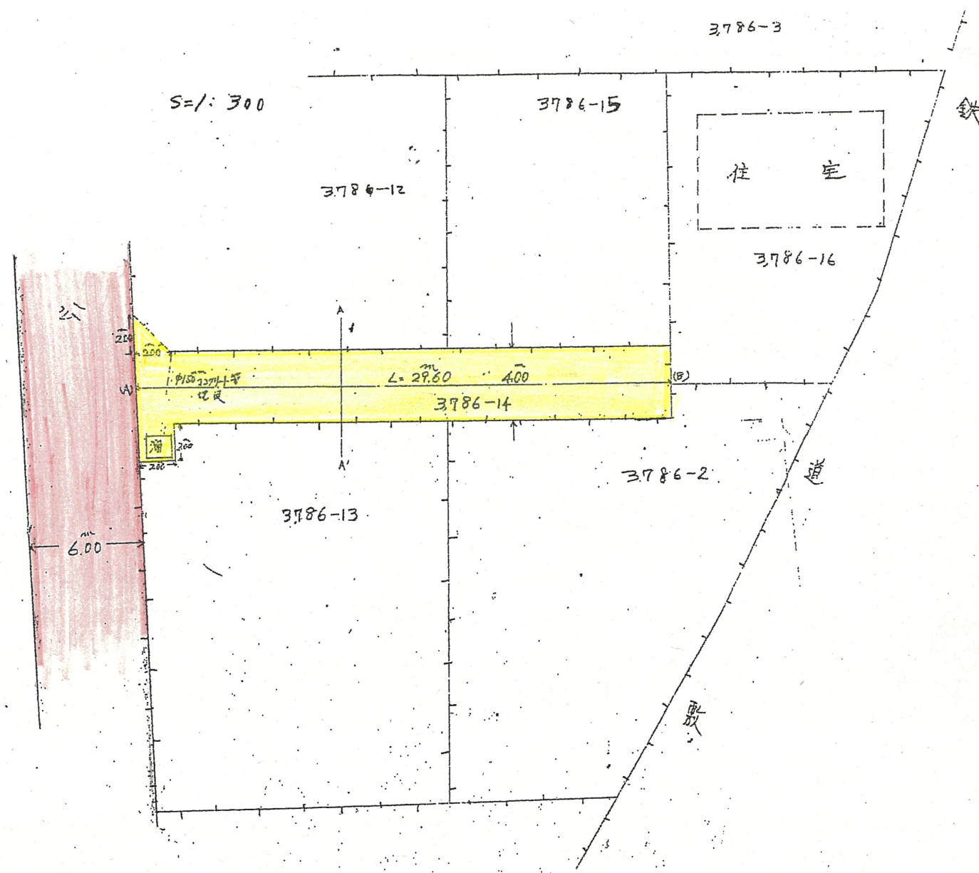
平面図 S = 1 / 300
