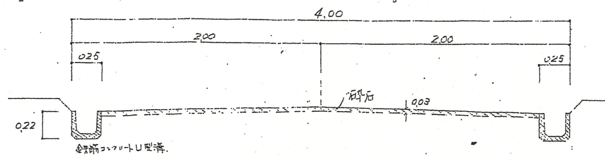
断面図 S = 1 / 30
