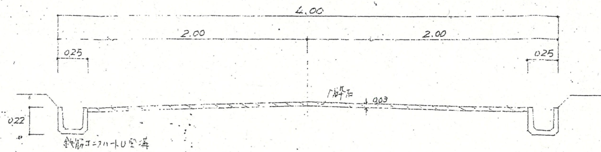
断面図 S = 1 / 30
