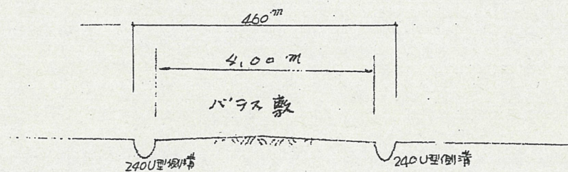
断面図 S=1/20
