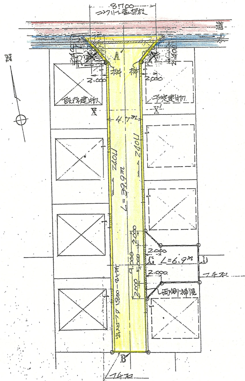
平 面 図 S = 1 / 300
