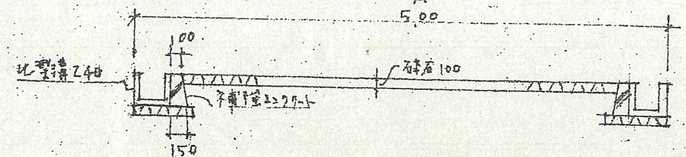
断面図 S = 1/50
