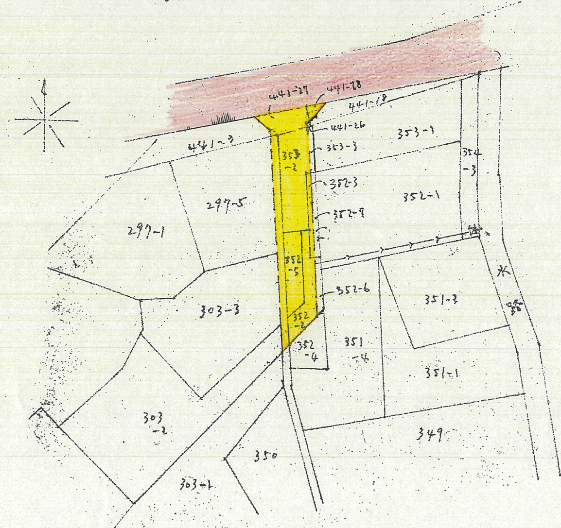
公図写 S = 1/500
