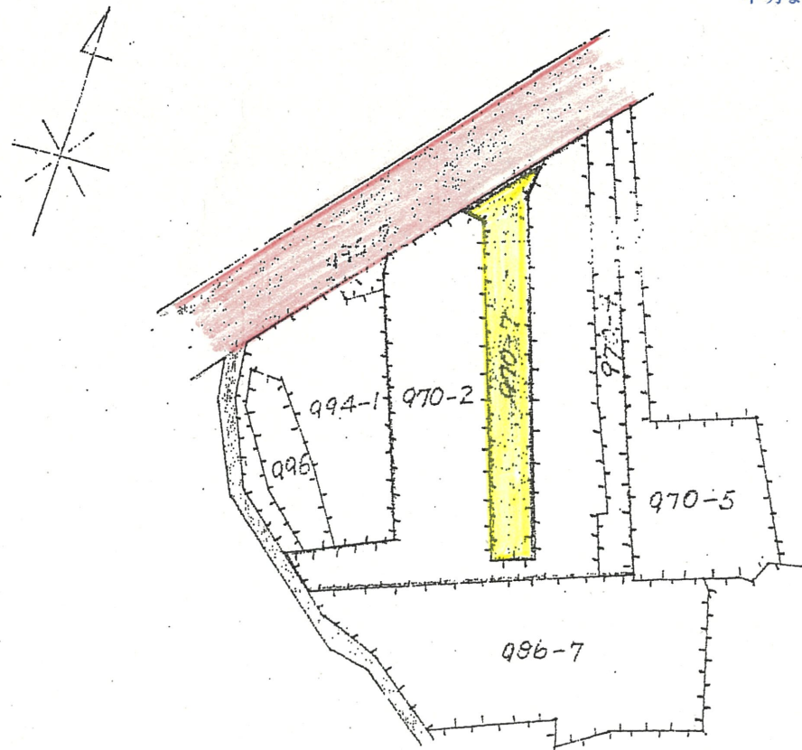
公 図 写 S = 1 / 600
