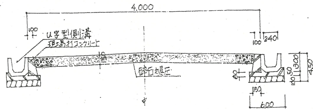
断 面 図 S = 1 / 40
