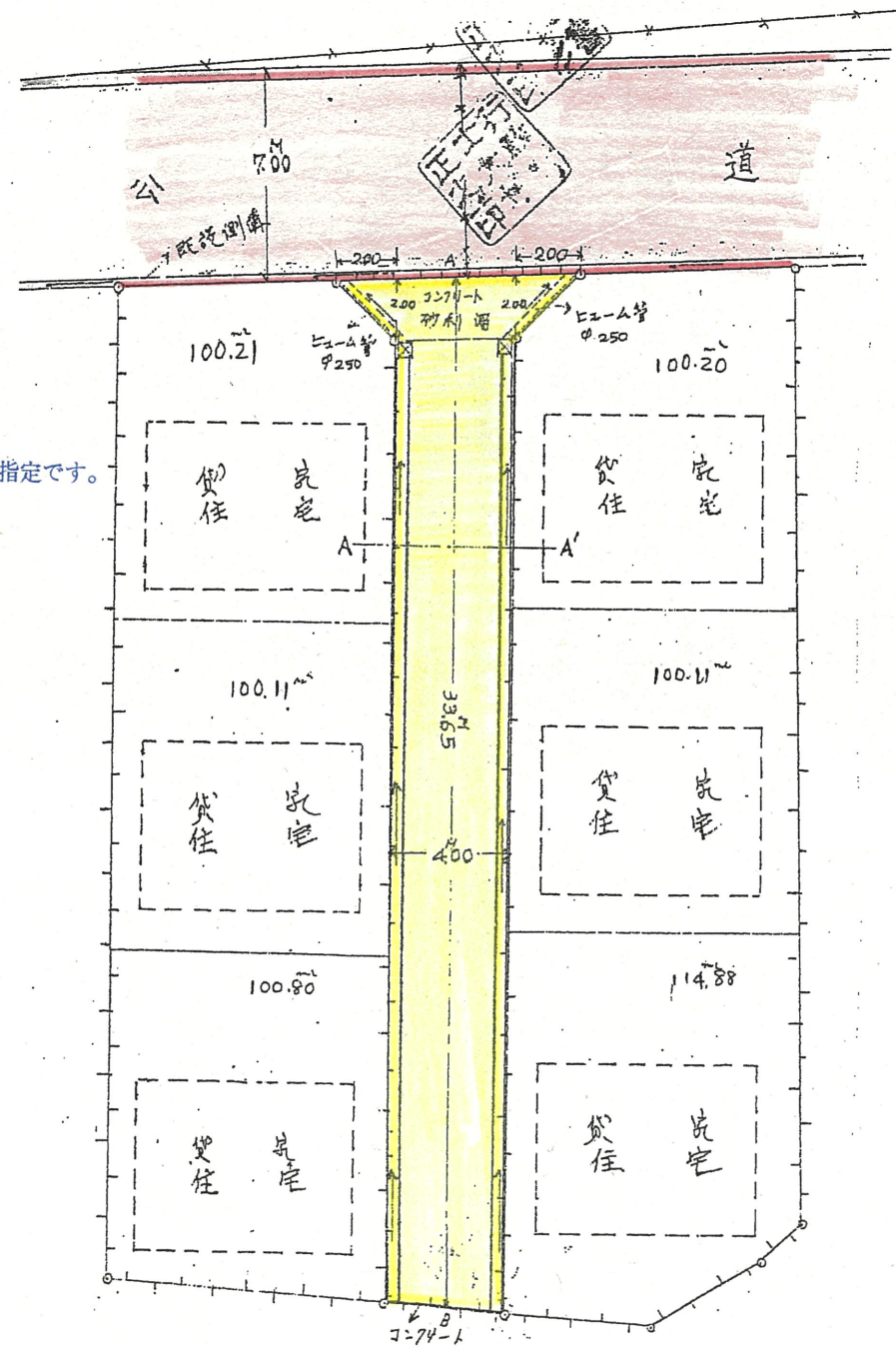
平面図 S = 1 / 250
