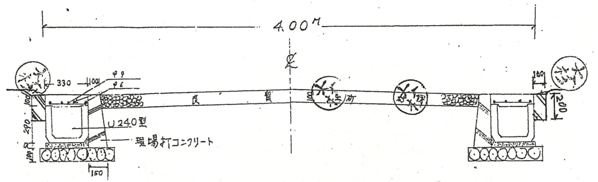
断面図 S = 1 / 30
