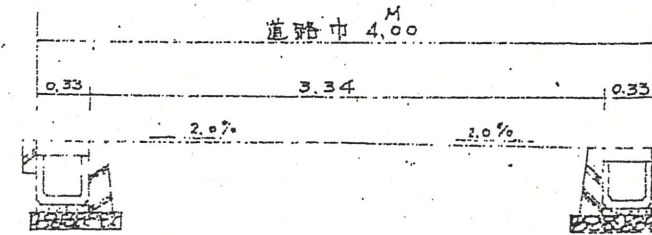
断面図 S=1/50
