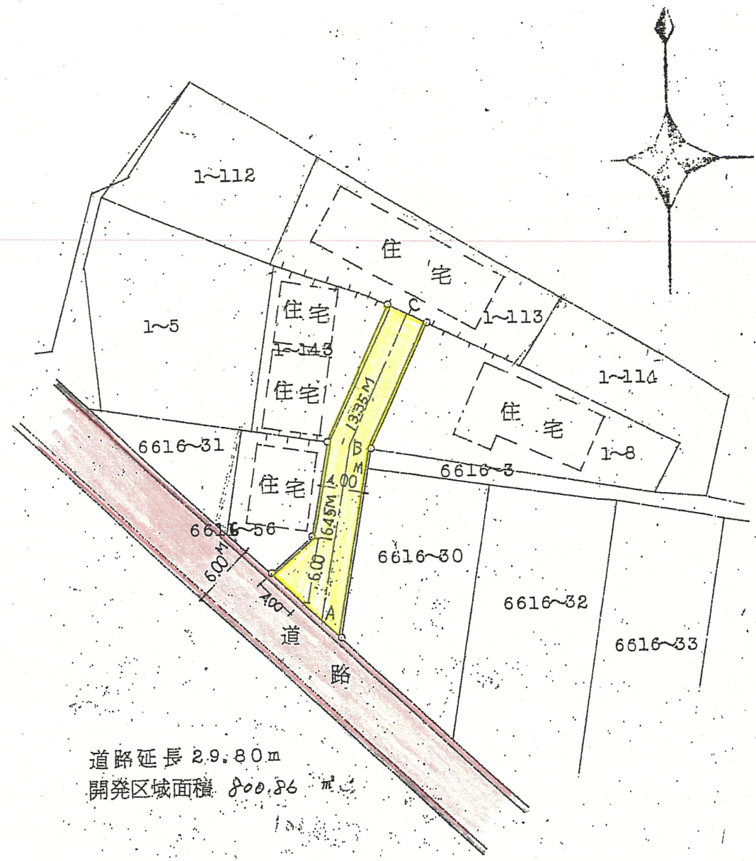
平面図 S = 1 / 500
