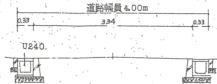
断面図 S = 1 / 50
