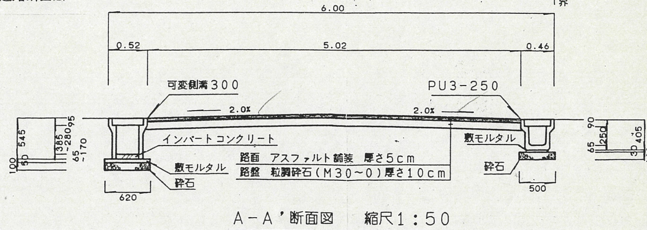
道路断面図
