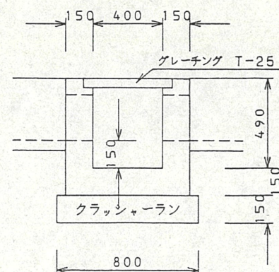
集水枘 1:50
