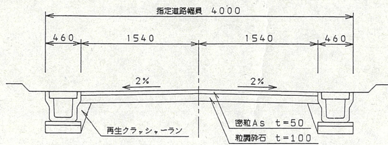
A-A断面図 1:50
