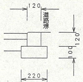
B-B断面図 1:20
