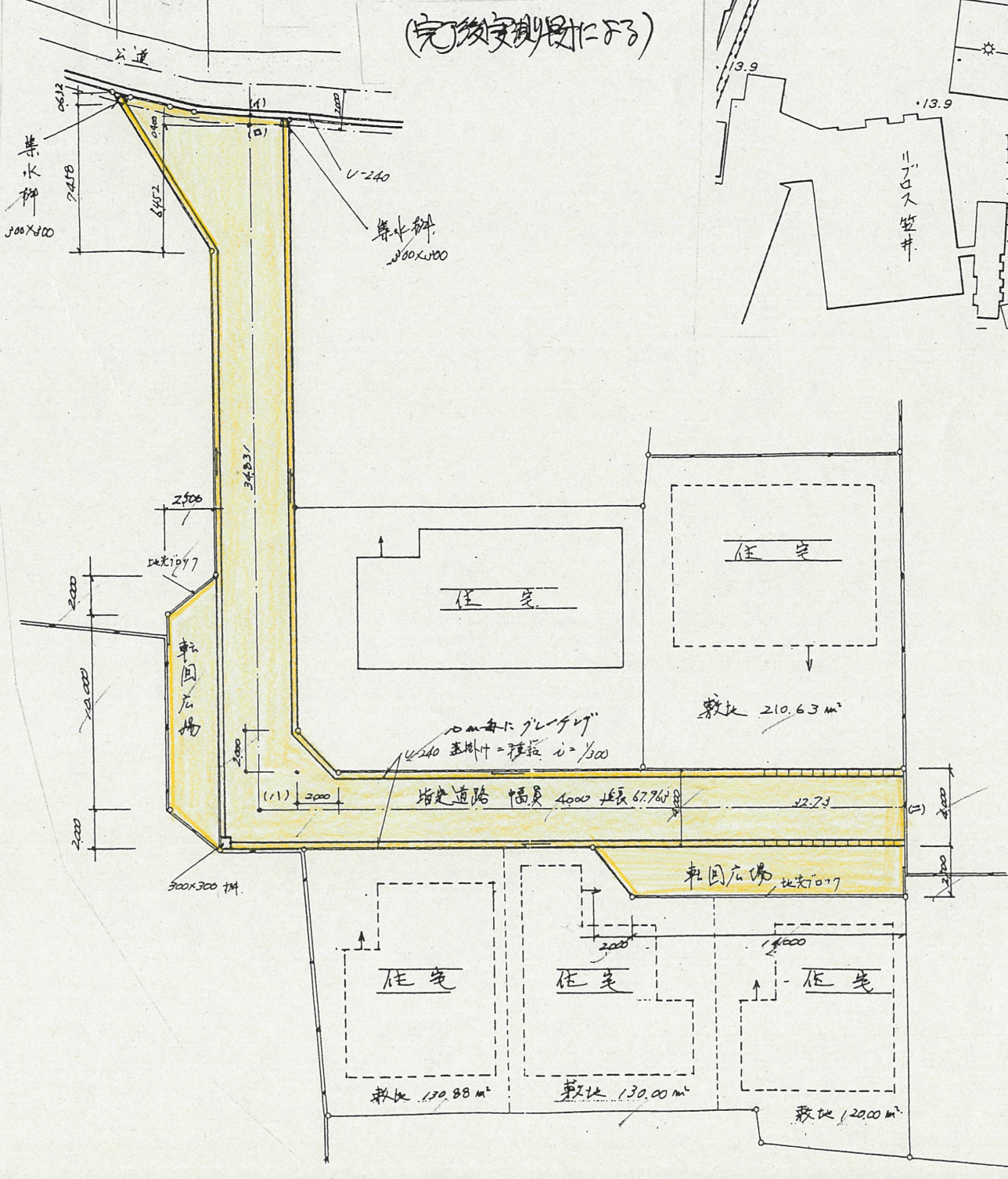
実測図 1/500
