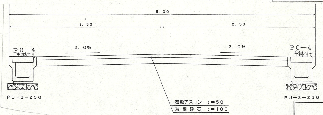
道路断面図 S = 1 / 30
