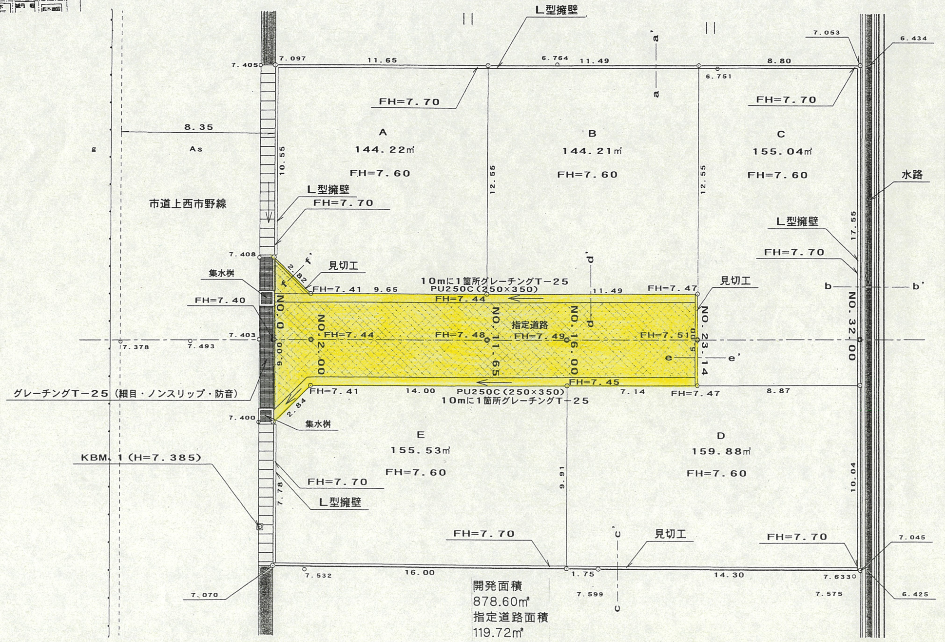
実測図 縮尺：1/200
