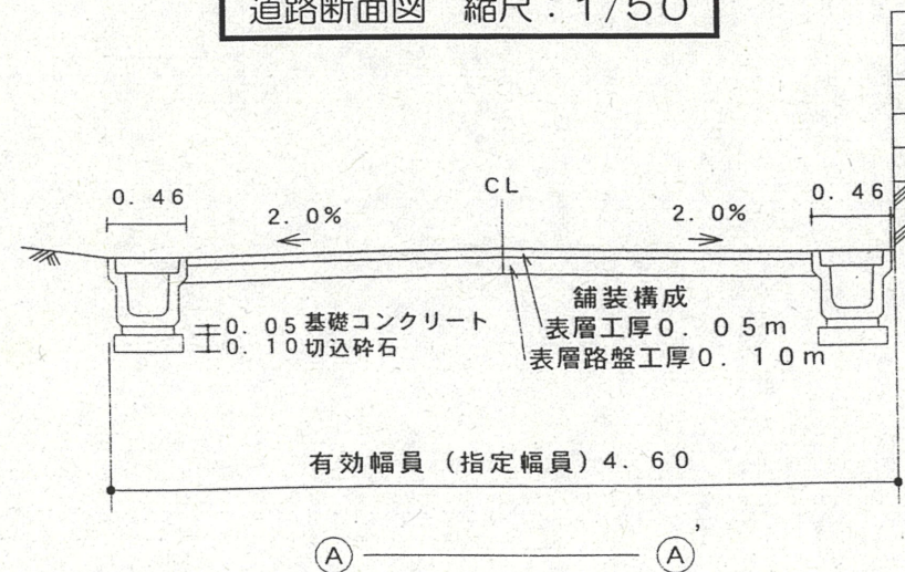
道路断面図 縮尺: 1/50
