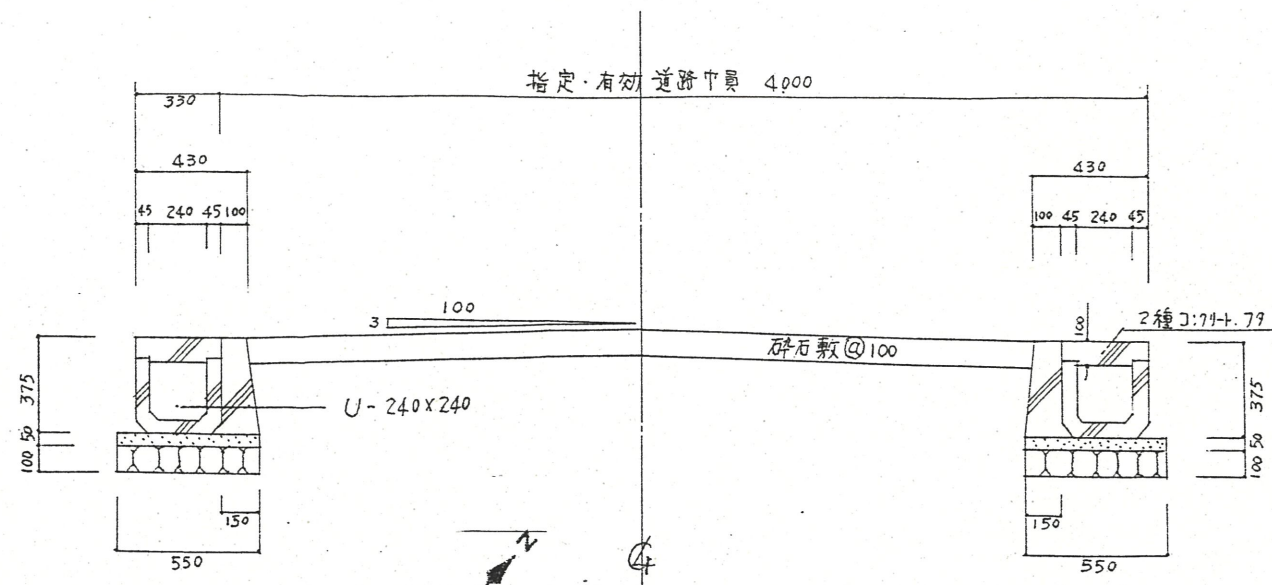
2 断面図 S: 1/30
