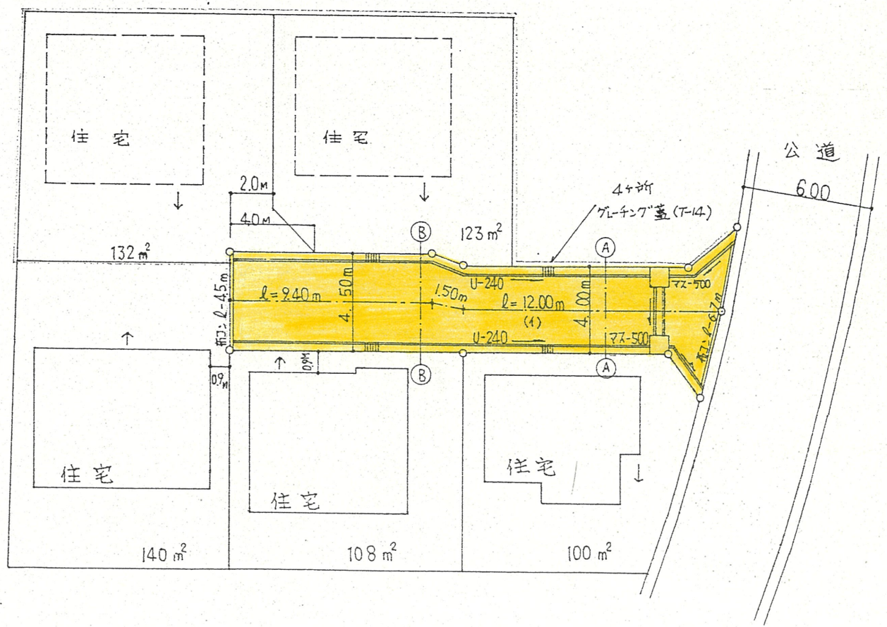
実測図 S=1:250
