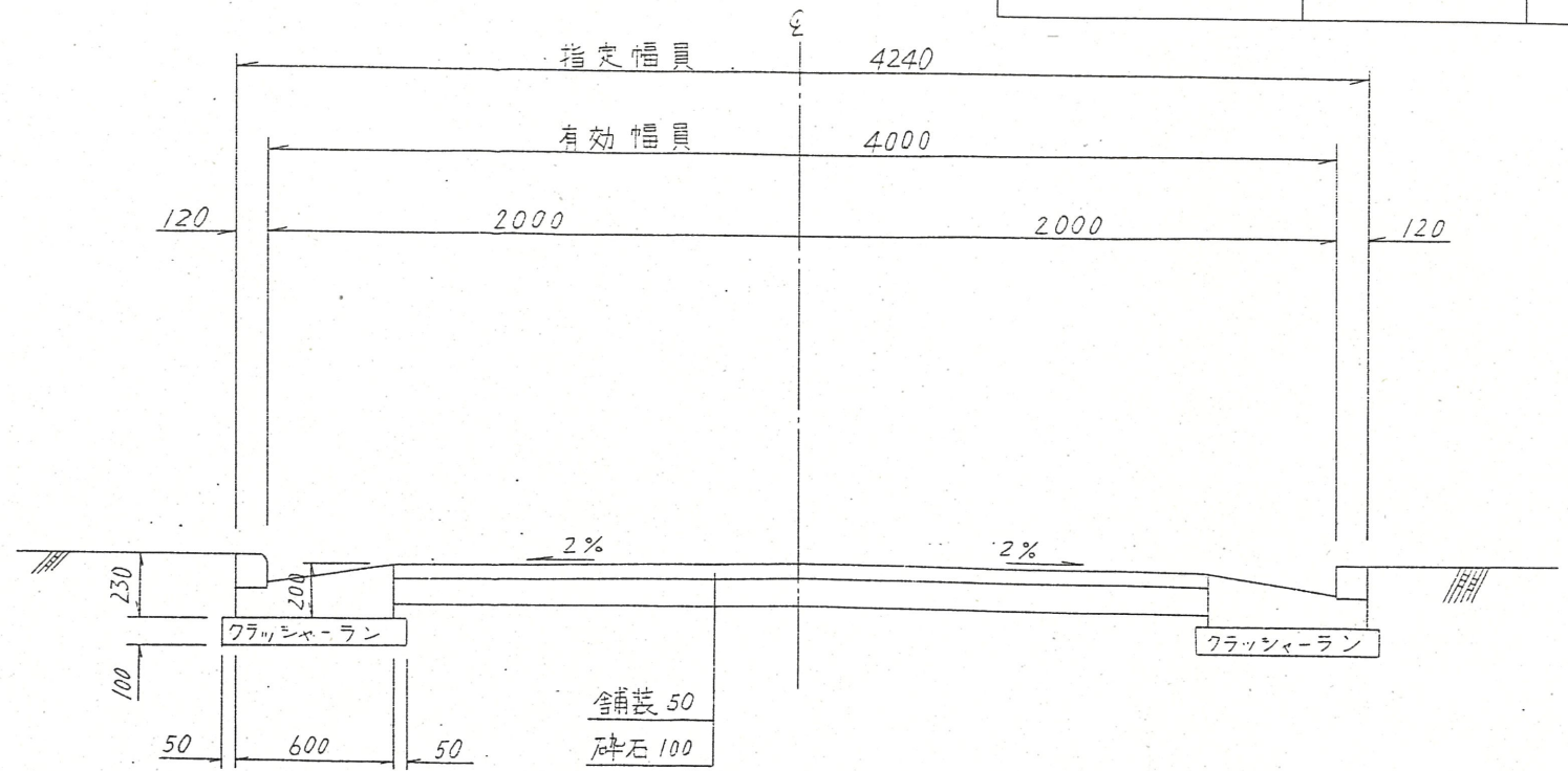
2 断面図 S = 1/30
