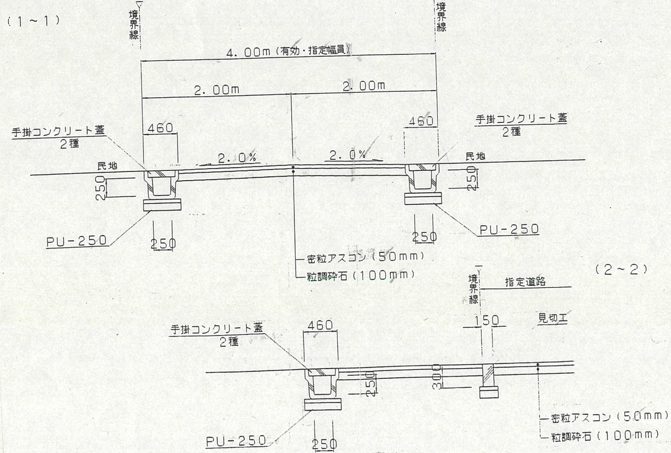
道路断面図 S=1:50
