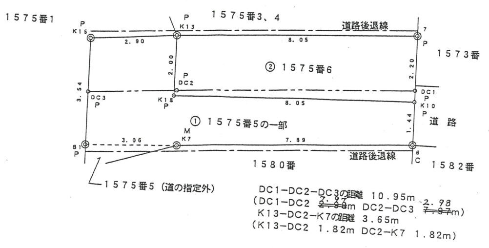
実測図 1/125
