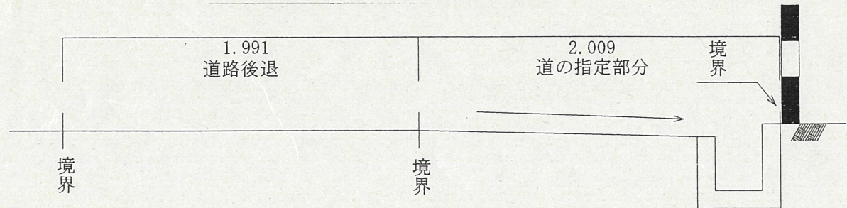
道路断面図 縮尺：1/30
