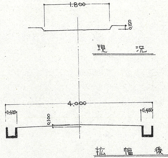
断面図 1/50
