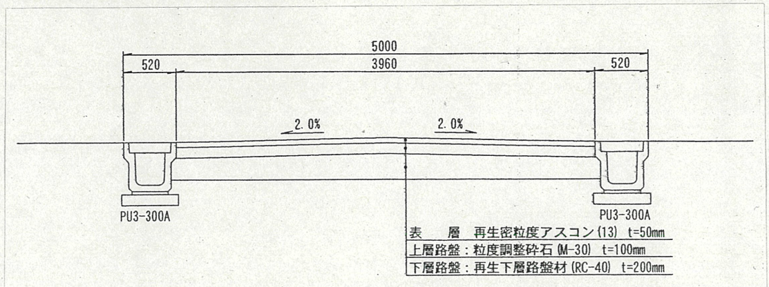
道路断面図 縮尺:1/50
