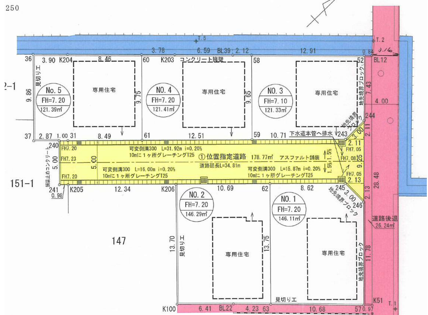
実測図 縮尺:1/250
