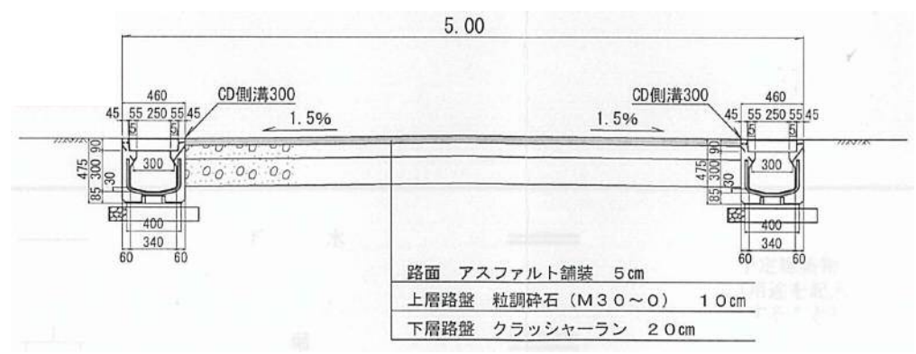
断面図 縮尺:1/50
