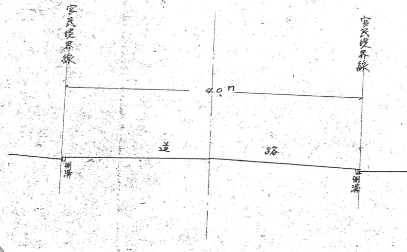
断面図
