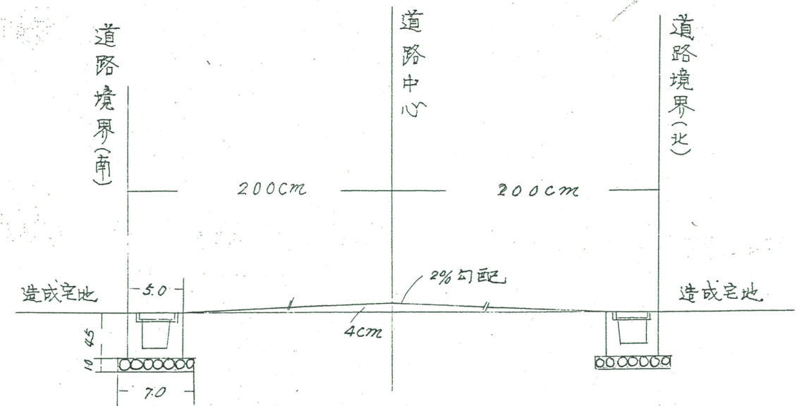
断面図
