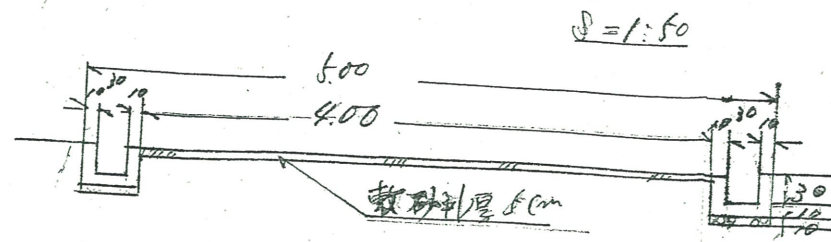
断面図 (B)
