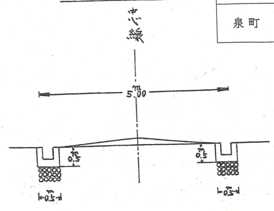
ABC断面図
