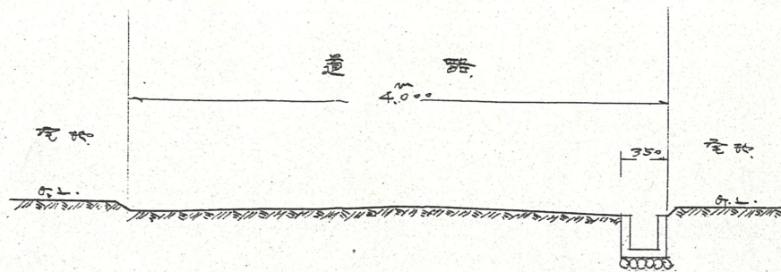
断面図 1/50
