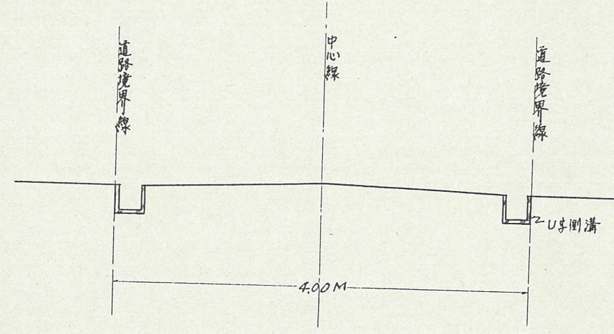
断面図 1/500
