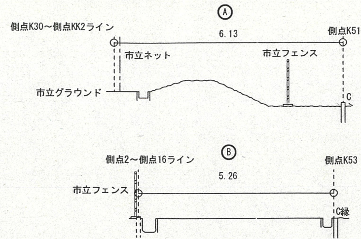
道路断面図 縮尺: 1/100
