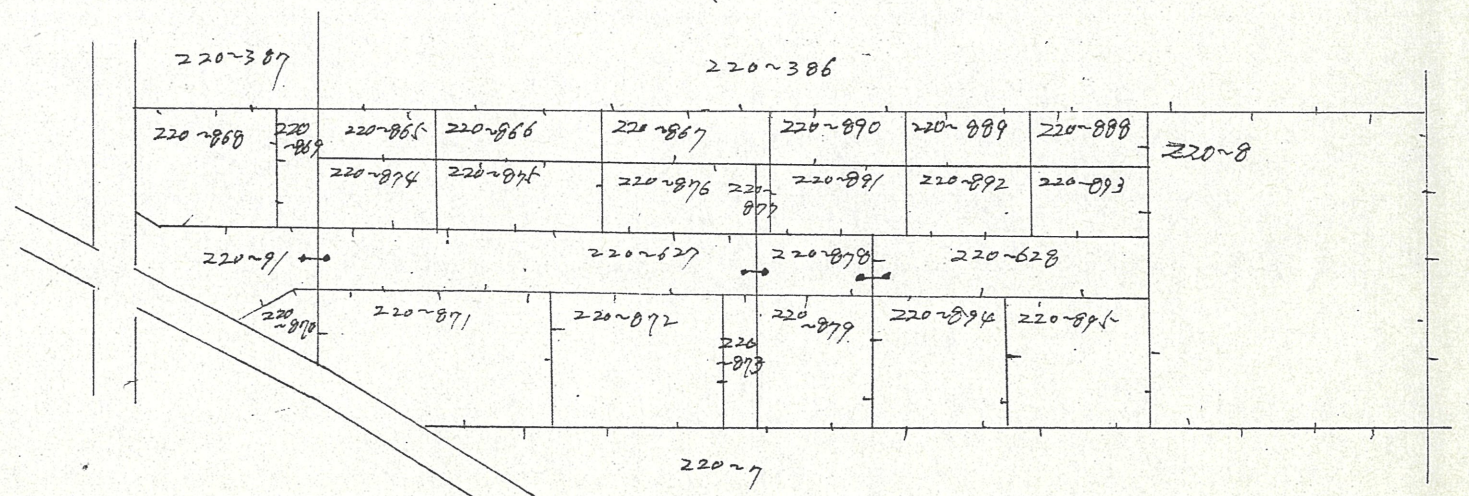
公図写 1/600
