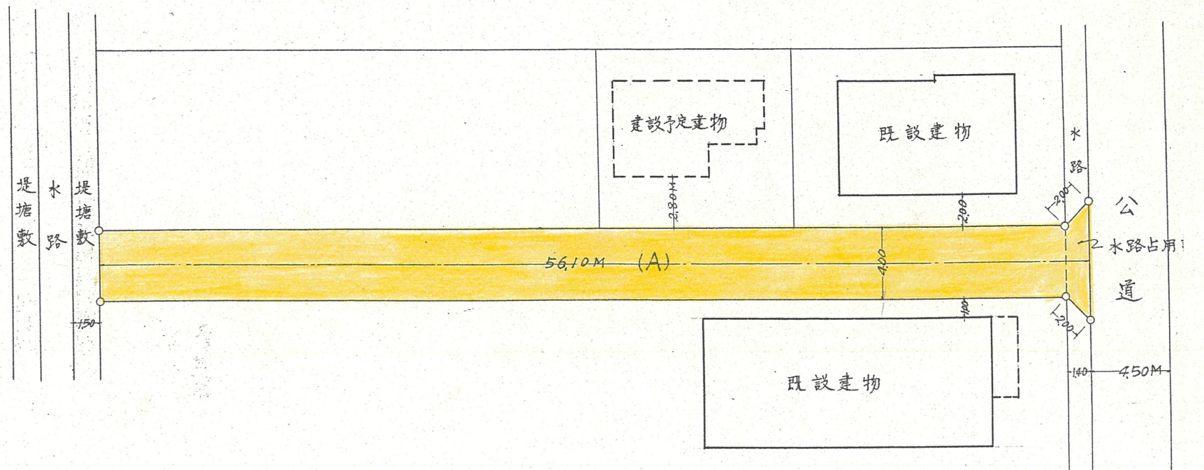
実測図 1/300
