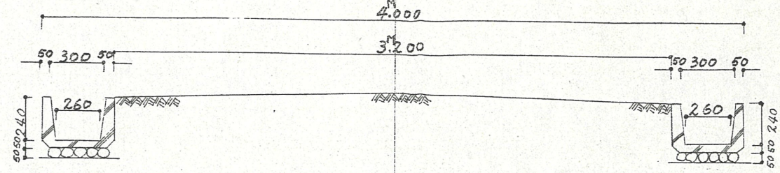
申請道路及び取合道路共通断面図 1/30
