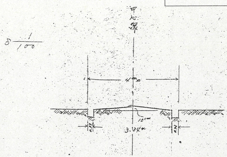
断面図
