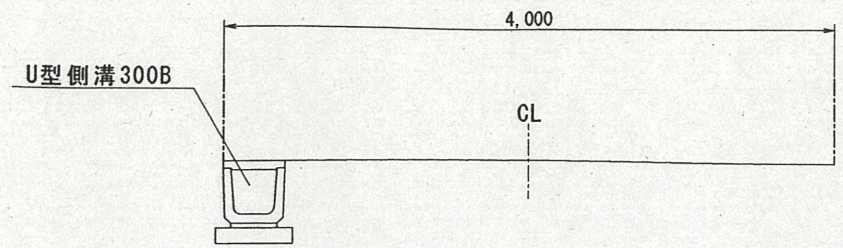
実測図 縮尺：1/300
