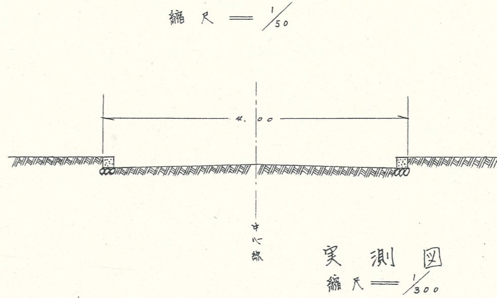
断面図
