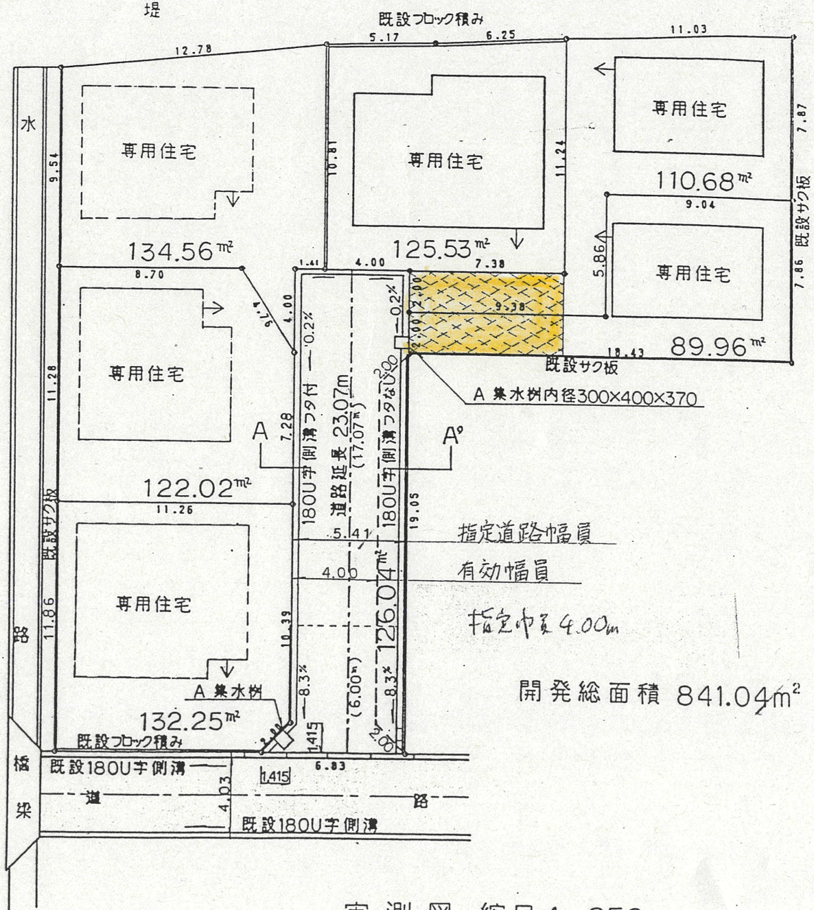
実測図 縮尺 1:250
