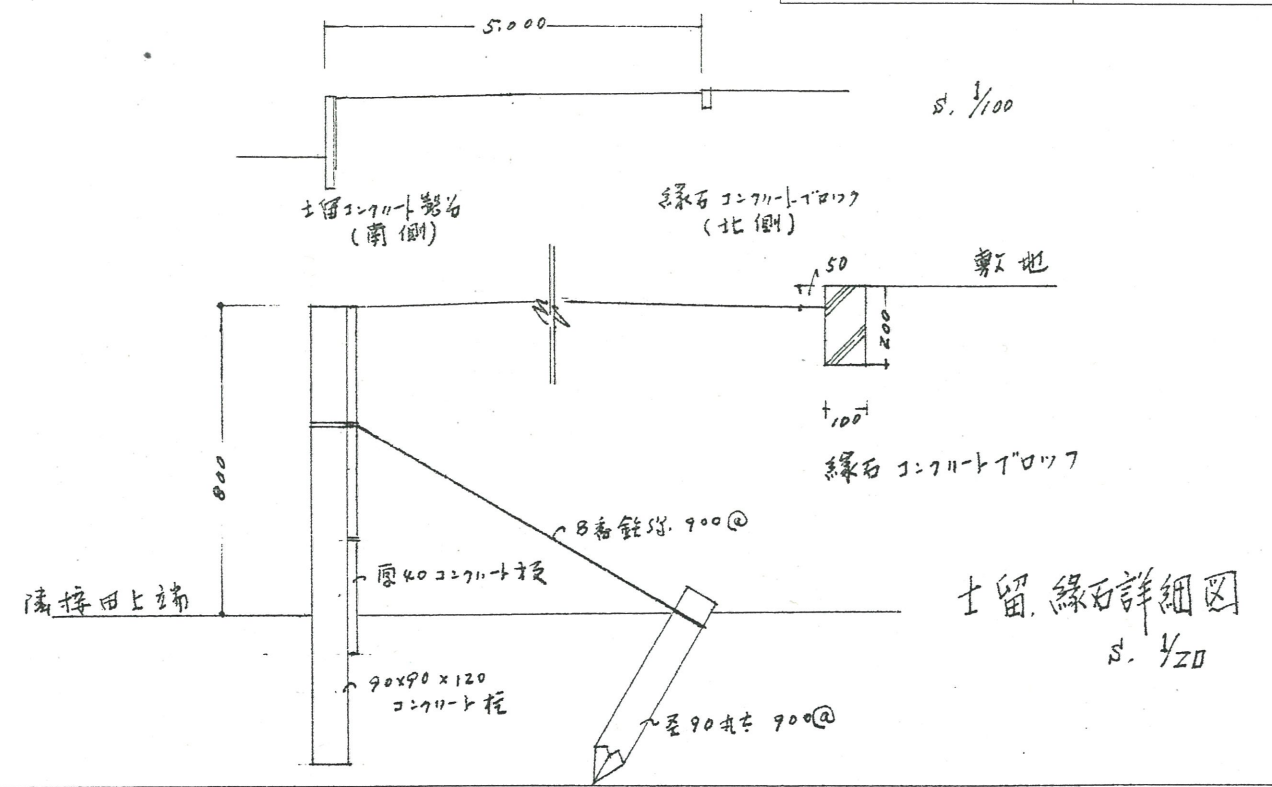
断面図
