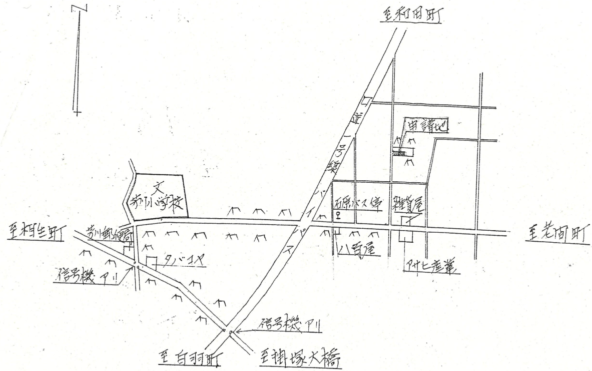
地籍図 (実測図及び公図写) 5L, 1/500
