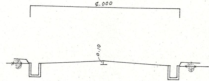
断面図 \frac{1}{50}
